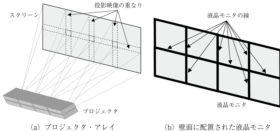
図 2 Tiled ディスプレイ
