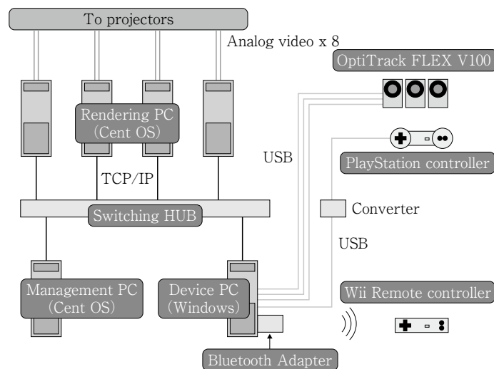
図5 システム構成
