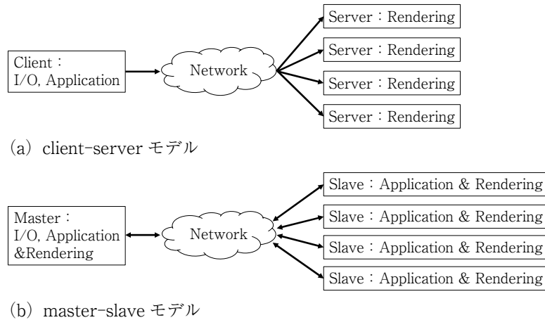
図3 分散レンダリングのモデル
